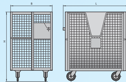
Open metalen rolcontainer 2400 liter
